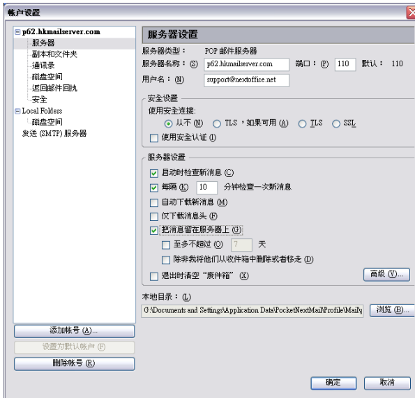
圖 24 帳號設定
