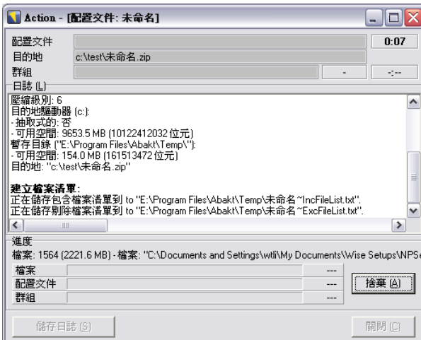
圖 33 執行動作
