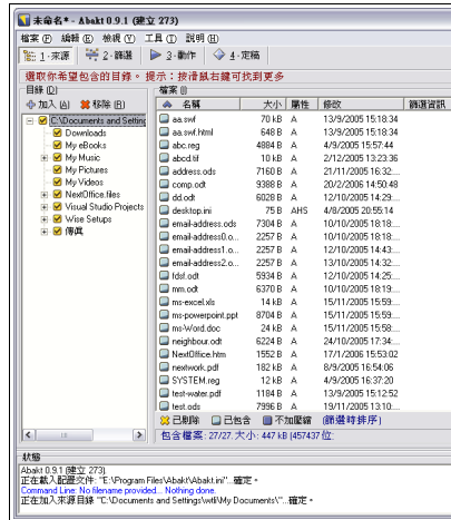
圖 29 選取來源
