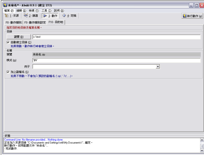
圖 32 選取目的地
