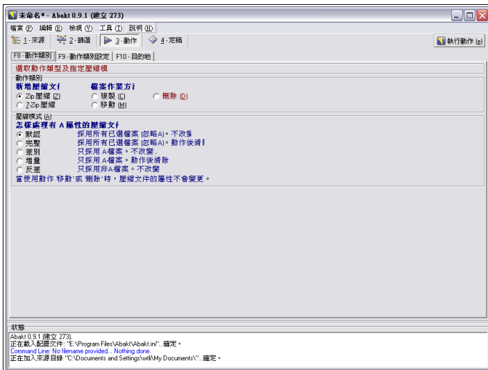
圖 31 選取其他的動作
