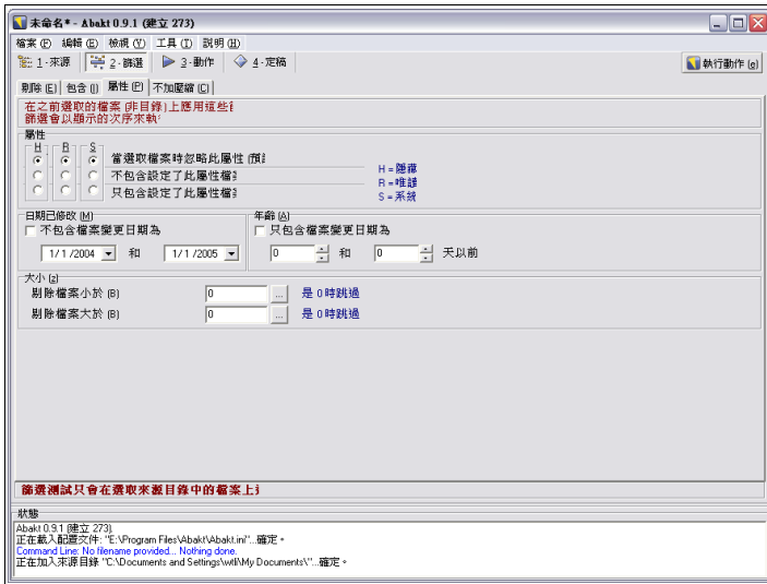
圖 30 定義篩選
